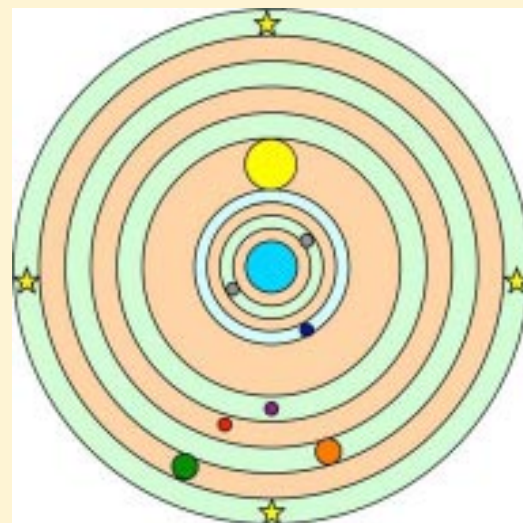
Model de Ptolomeu: en aquest model, la Terra (color blau) ocupa el centre de l'univers en el qual es manté, mentre la resta dels planetes i el Sol (color groc) l'orbiten dins d'unes esferes.
