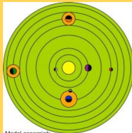
Model copernicà: Copèrnic situa el sol (color groc) al centre de l'univers i els planetes al seu voltant. La Lluna (color gris) la situa en òrbita de la Terra (color Blau). També situa llunes orbitant Júpiter.
